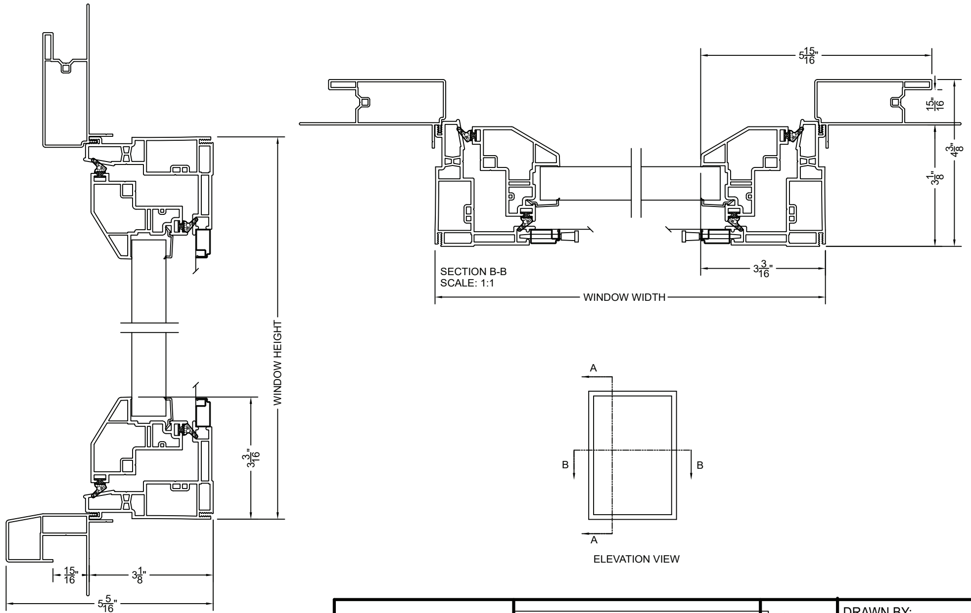
SECTION A-A SCALE: 1:1
